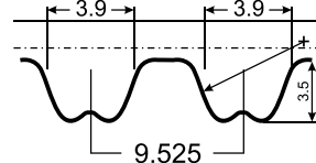
Профиль ремней ГРМ 2108-1006040 и 2112-1006040
